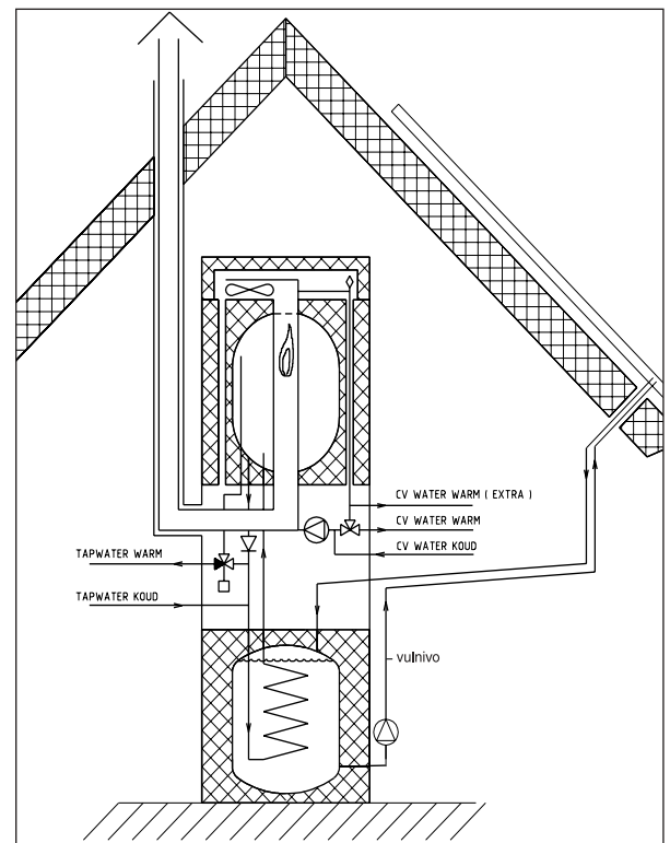
FIGUUR 2.1: PRINCIPEWERKING MULTISOLAR
